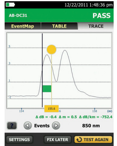
超短事件和衰减死区
