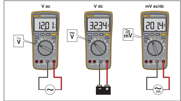
图 1. 测量交流和直流电压
