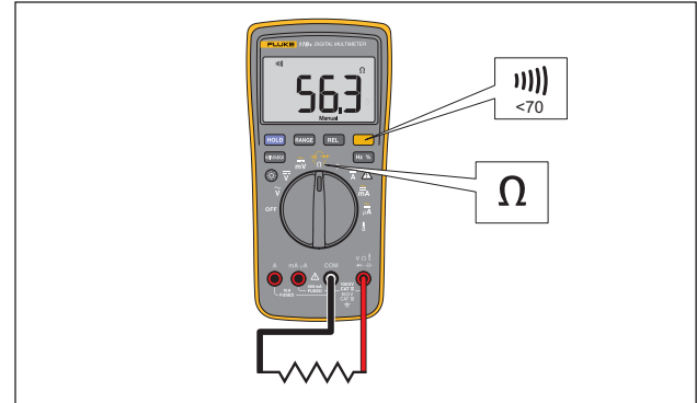
图 3. 测量电阻/通断性
