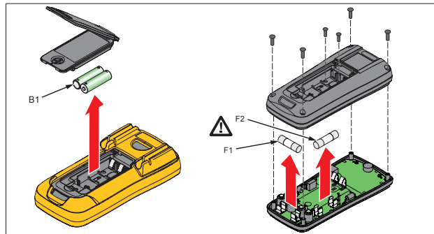
图 5. 更换电池和保险丝
